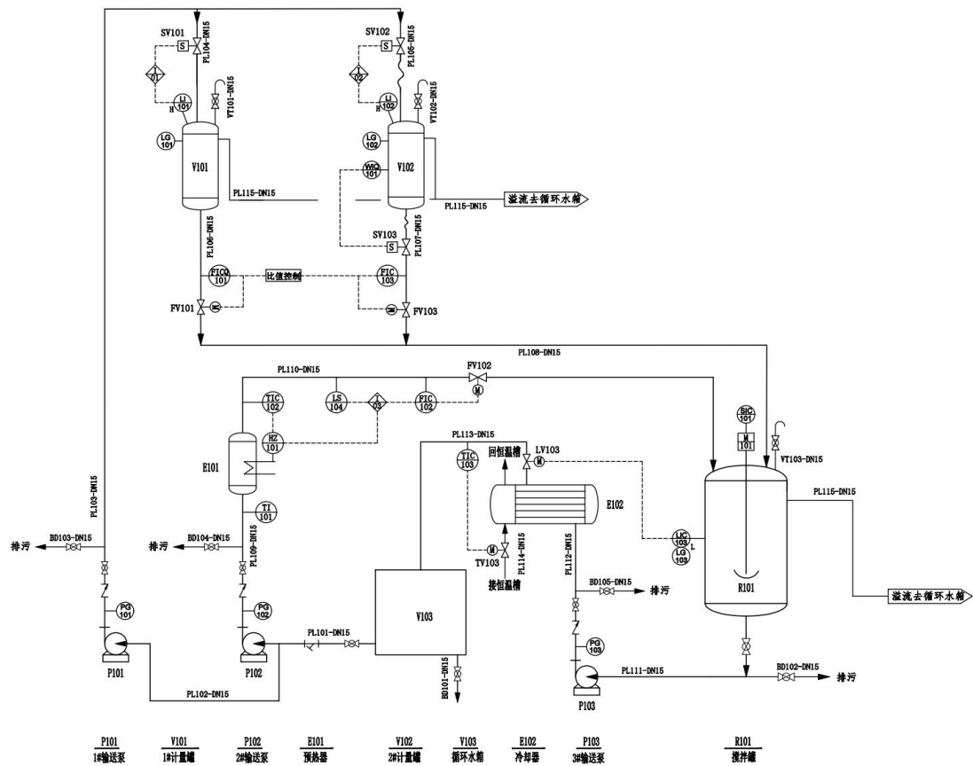
图 2 装置流程图 (仅供参考)
